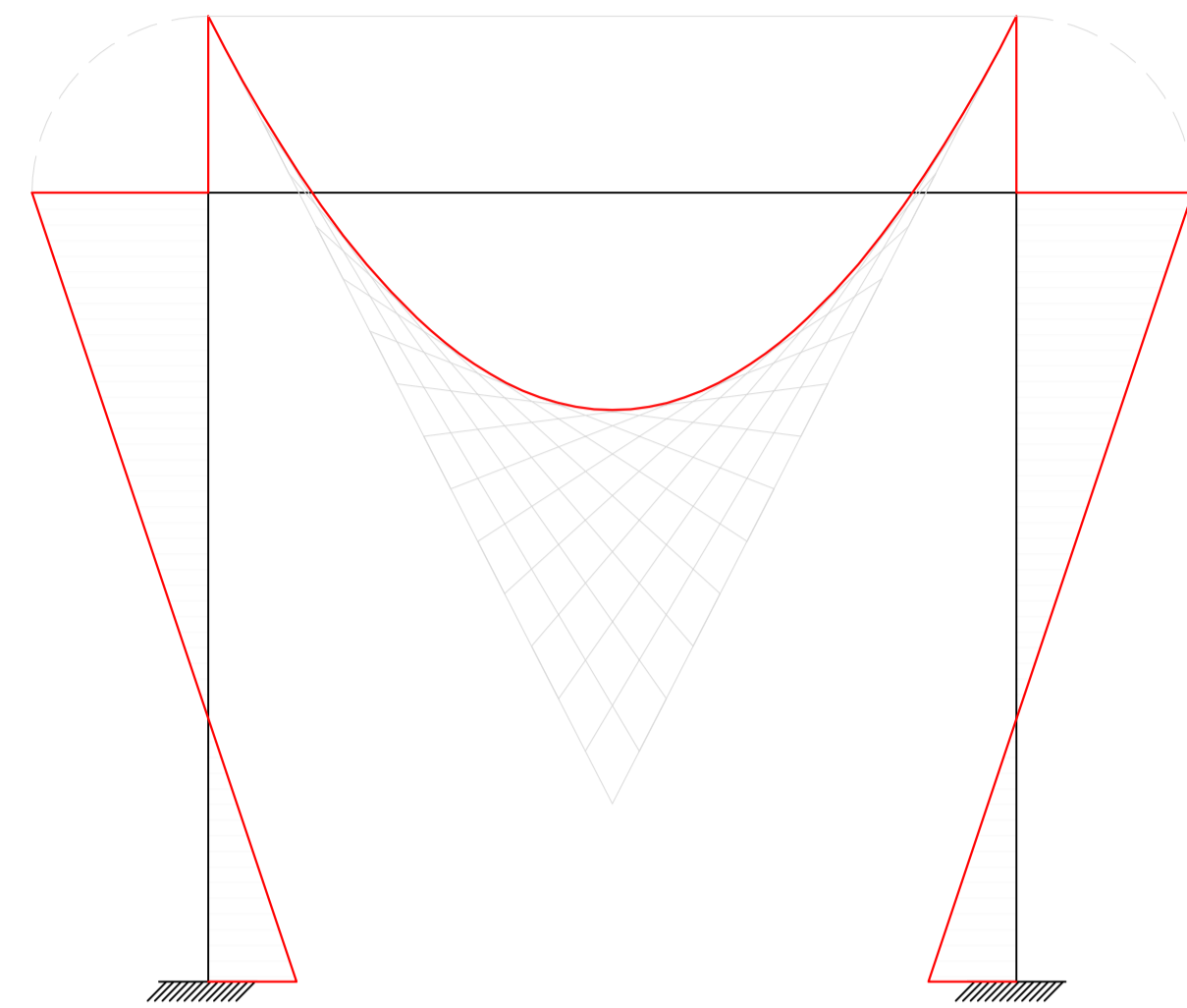
Diagramma Momento Flettente SCALA 1cm=20KN
